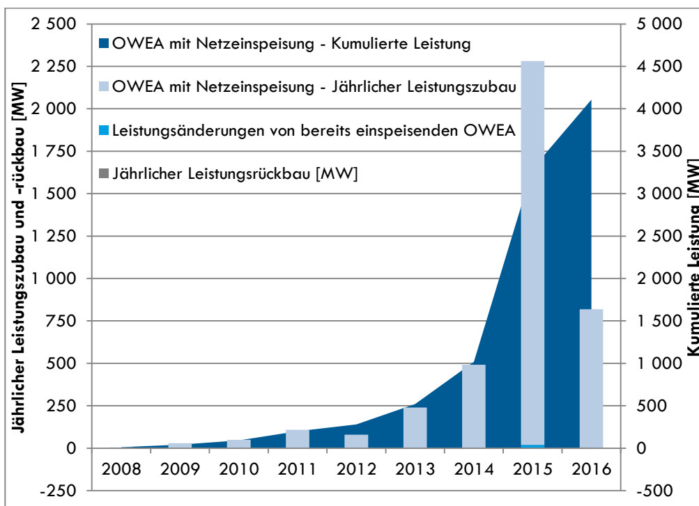
Abbildung 1: Entwicklung der Offshore-Windenergie in Deutschland (Kapazität der OWEA mit Netzeinspeisung), Stand 31.12.2016
