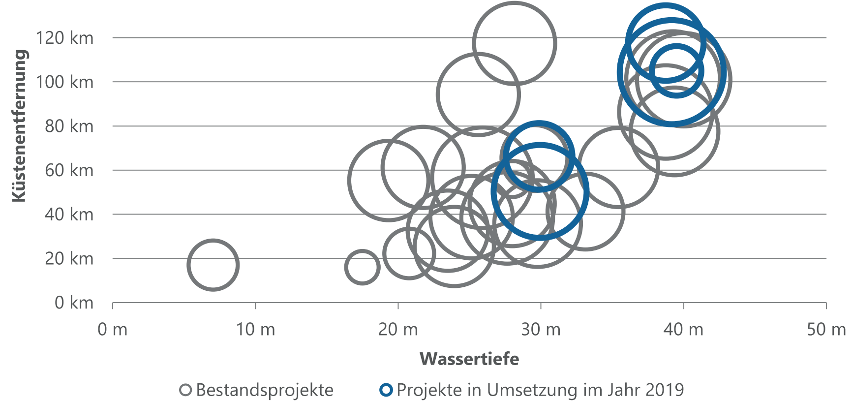
Wassertiefe und Küstenentfernung von Bestandsprojekten und Projekten in der Umsetzung
