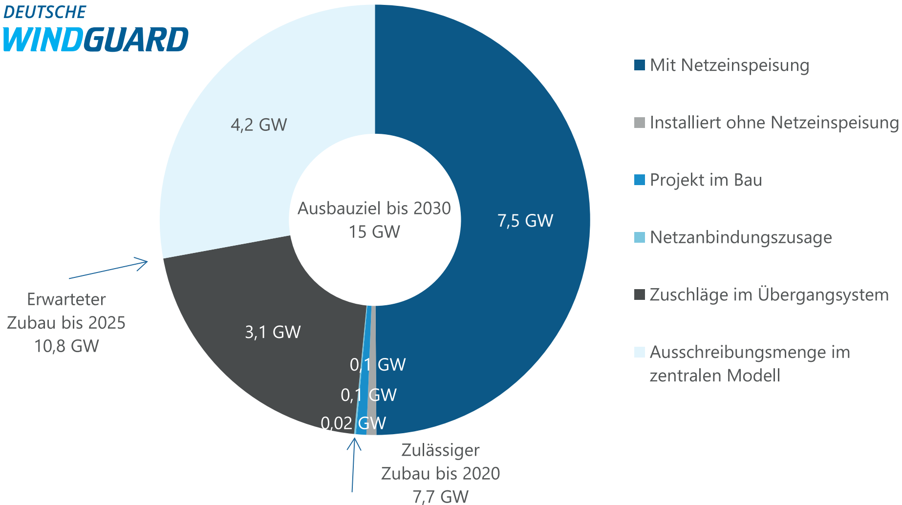
Entwicklungsstatus der Offshore-Leistung mit erwartetem Zubau bis 2030
